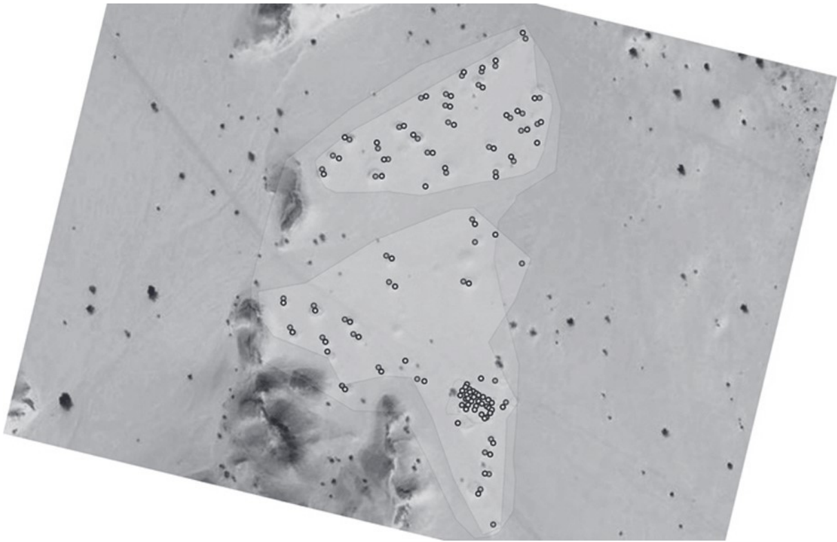
Abb. 4: Friedhof aus Tumuli und box graves (Sites W.A.D.I. 3712/3713) mit Ergebnissen der Fernerkundung und des Ground-checks.
