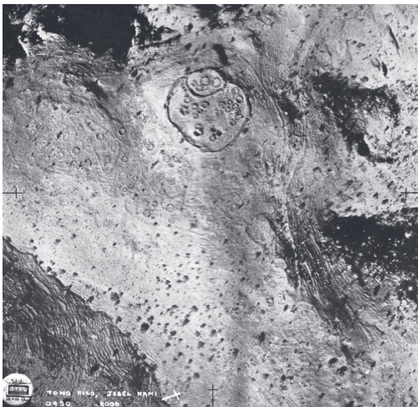
Abb. 1: Luftaufnahme der Royal Air Force vom 14.1.1936 zu kartographischen Zwecken, die spätmittelalterliche Ruinen am Jebel Nami (Darfur) zeigt (nach Arkell 1937, Plate IV)
