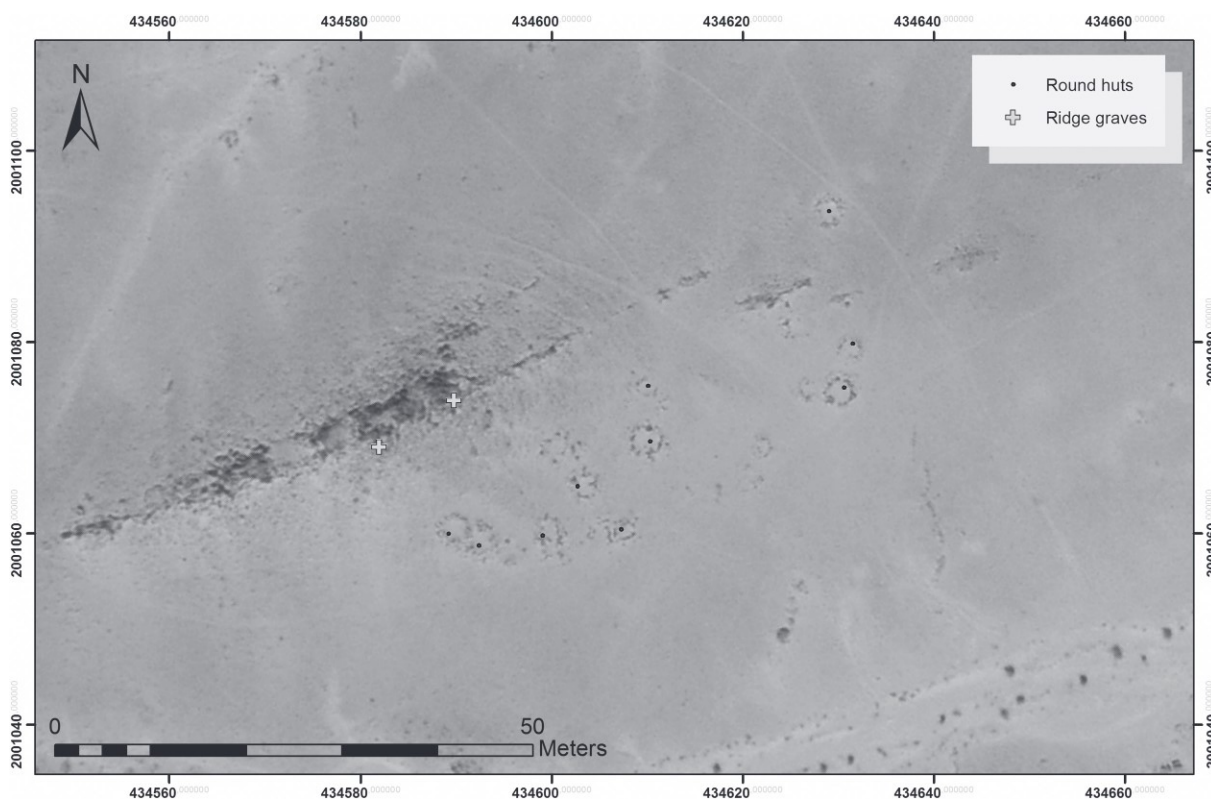
Abb. 6: Rundhüttengrundrisse im Luftbild (Site W.A.D.I. 19582)
